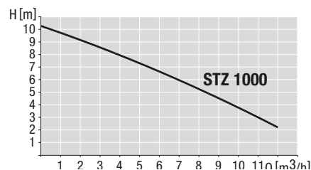
Abb. [5] Pumpenkennlinien
