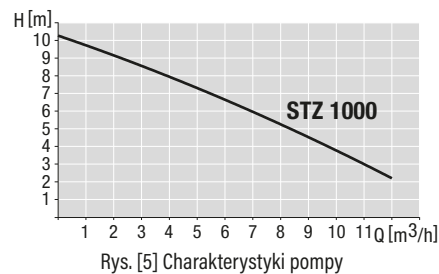
Rys. [5] Charakterystyki pompy
