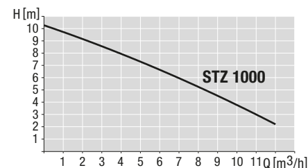
fig. [5] Courbes caractéristiques de la pompe
