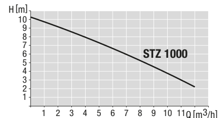
Afb. [5] Pompkarakteristiek
